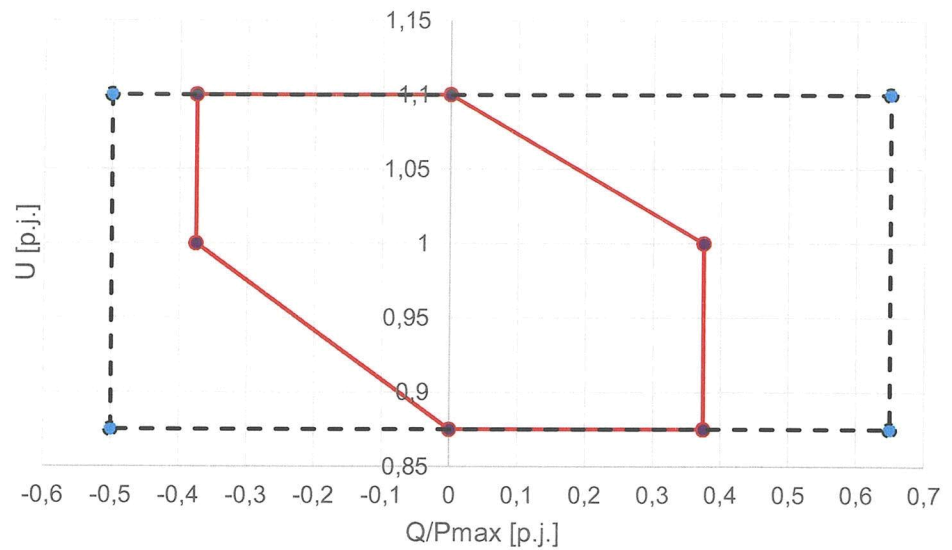
Obr. 1 Diagram dodávky jalového výkonu při maximální dodávce činného výkonu pro nesynchronní výrobní moduly kategorie D
