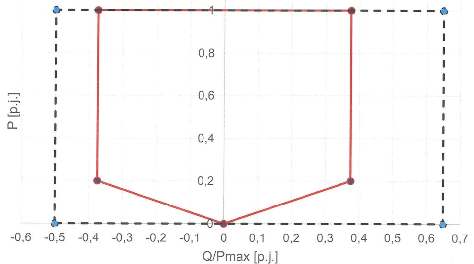
Obr. 3 Diagram dodávky jalového výkonu při nižší než maximální dodávce činného výkonu pro nesynchronní výrobní moduly kategorie D
